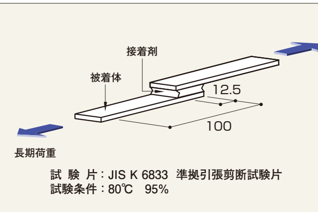
図-1 デッドロードストレス試験概要
