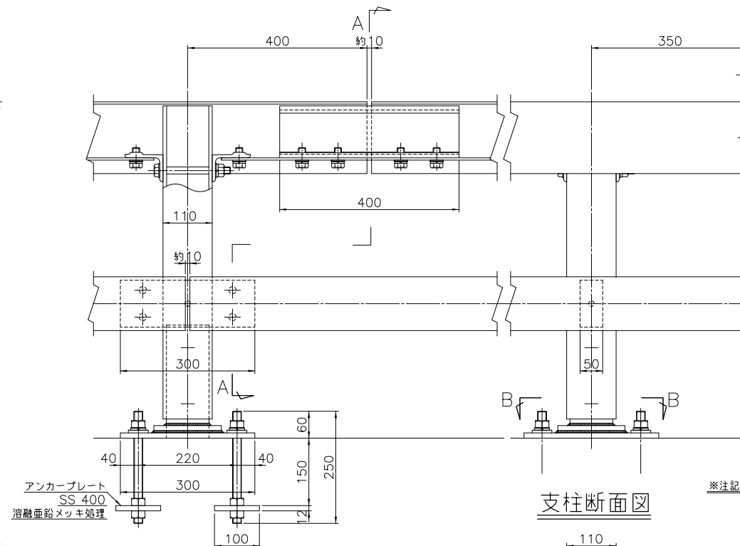
継手部
