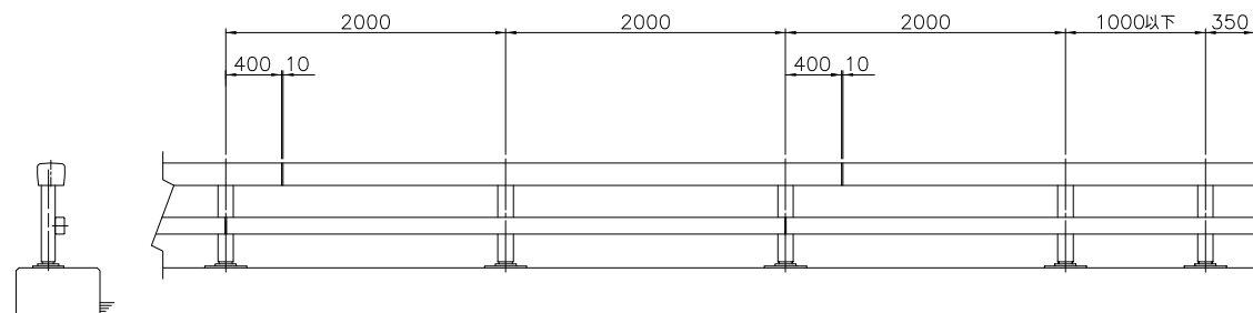
姿 図 S=1/30
