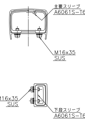
断面A-A
