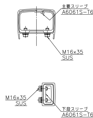
断面A-A
