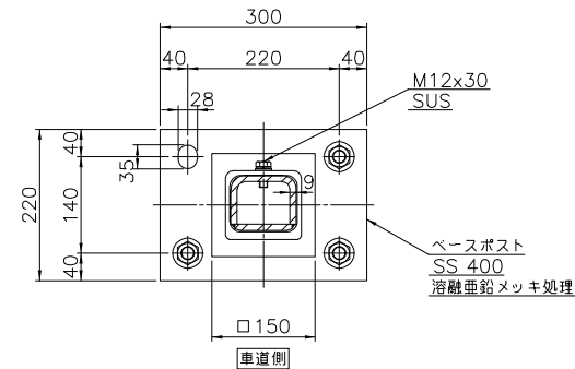
断面B-B
