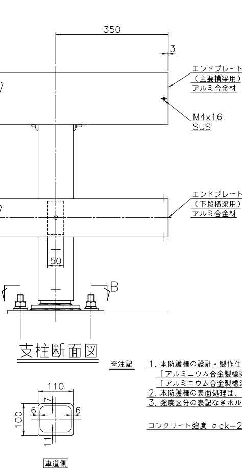
端 部
