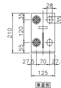
断面A-A
