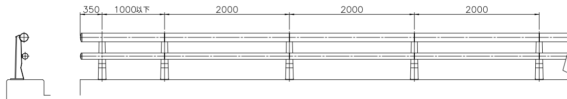
姿 図 S=1/30
