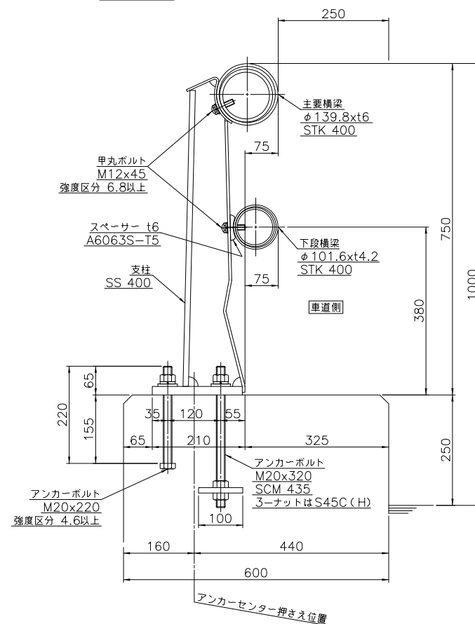
車両用防護柵取付詳細図 S=1/6 (種別 A)
