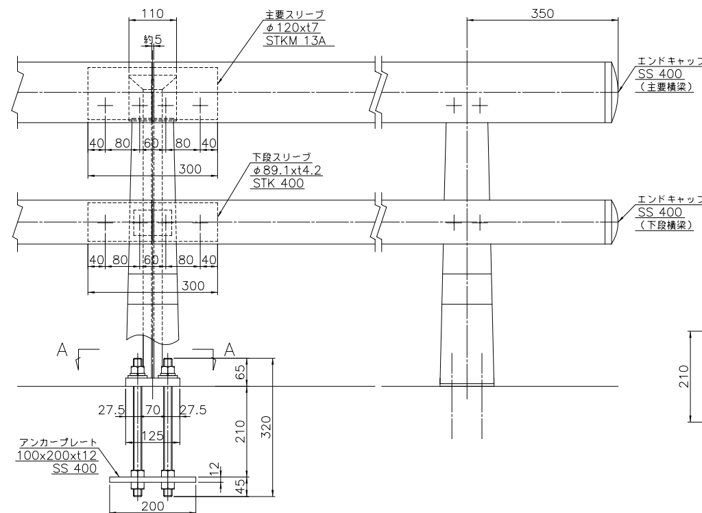
継手部
