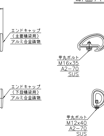
断面A-A
