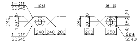
補強鉄筋図 S=1/20
