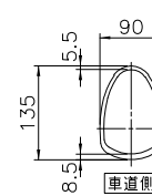
支柱断面図
