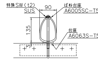
断面B-B
