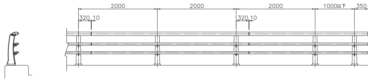
姿 図 S=1/30
