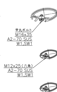
断面A-A
