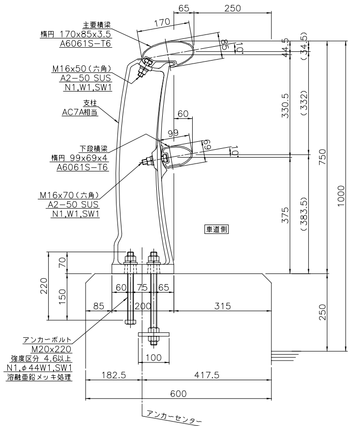
車両用防護柵取付詳細図 S=1/6
