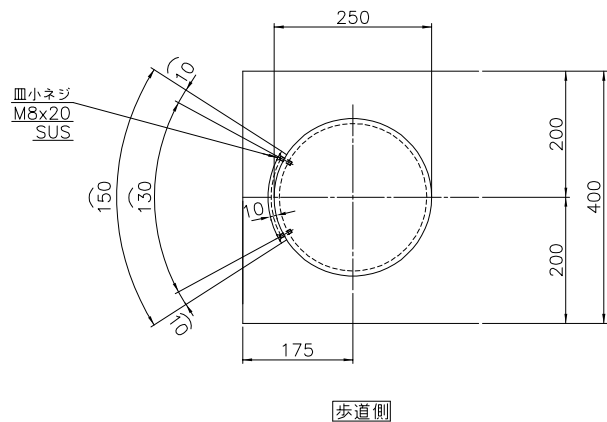
平面図 S=1/6
