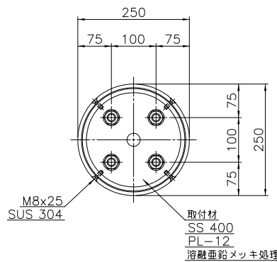
断面A-A
