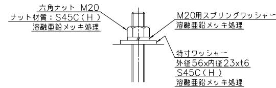
断面B-B
