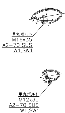
断面A-A
