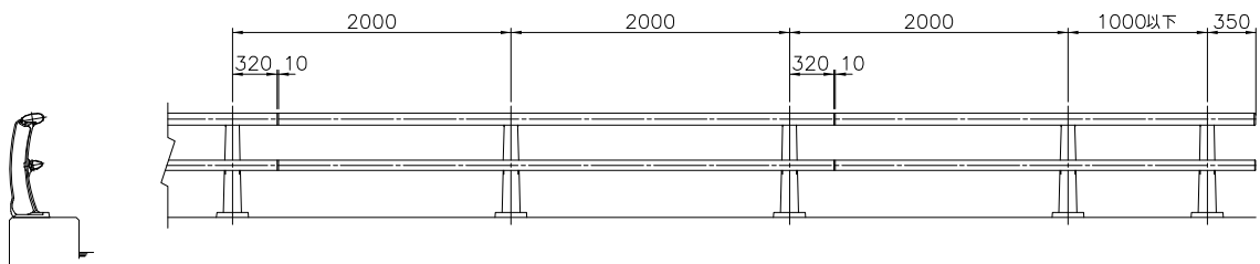
姿 図 S=1/30
