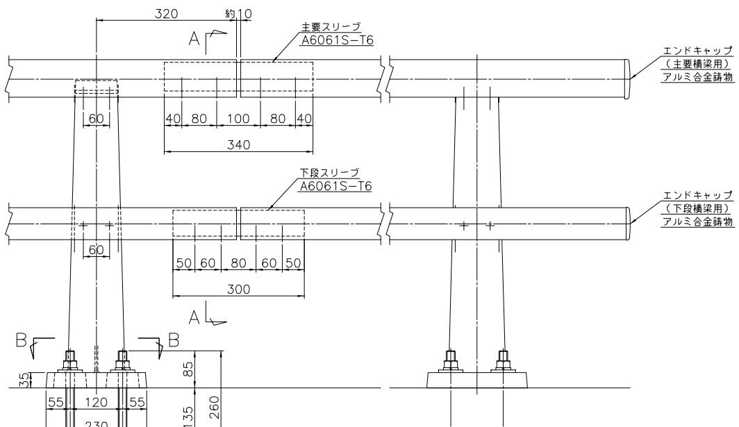
継手部
