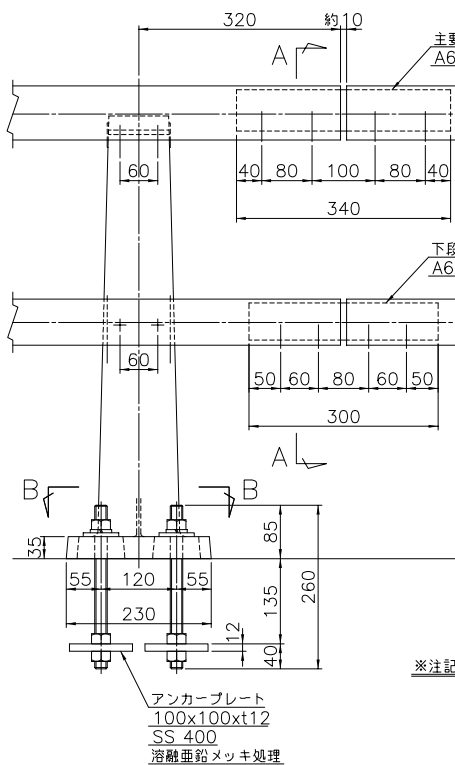
継手部
