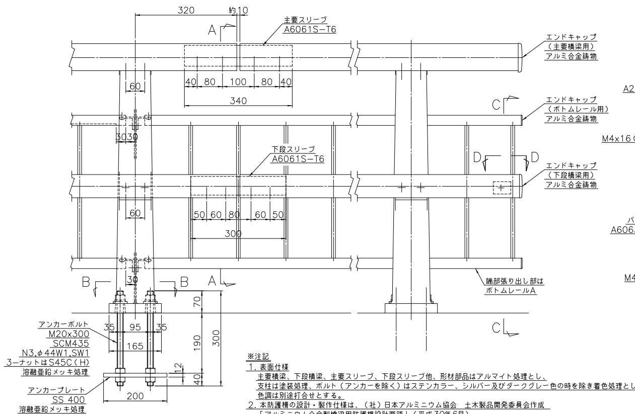
継手部
