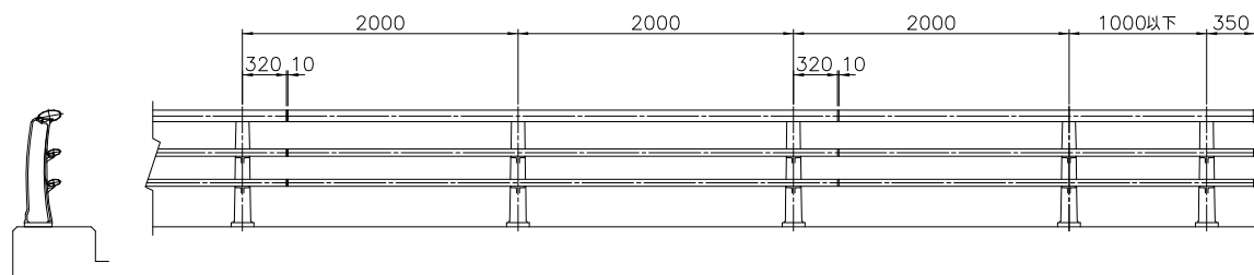
姿図 S=1/30
