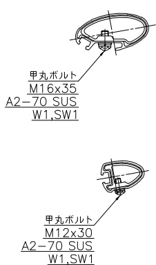
断面A-A
