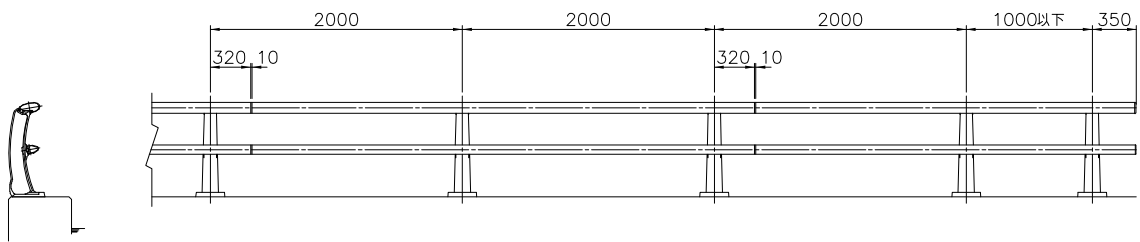
姿 図 S=1/30
