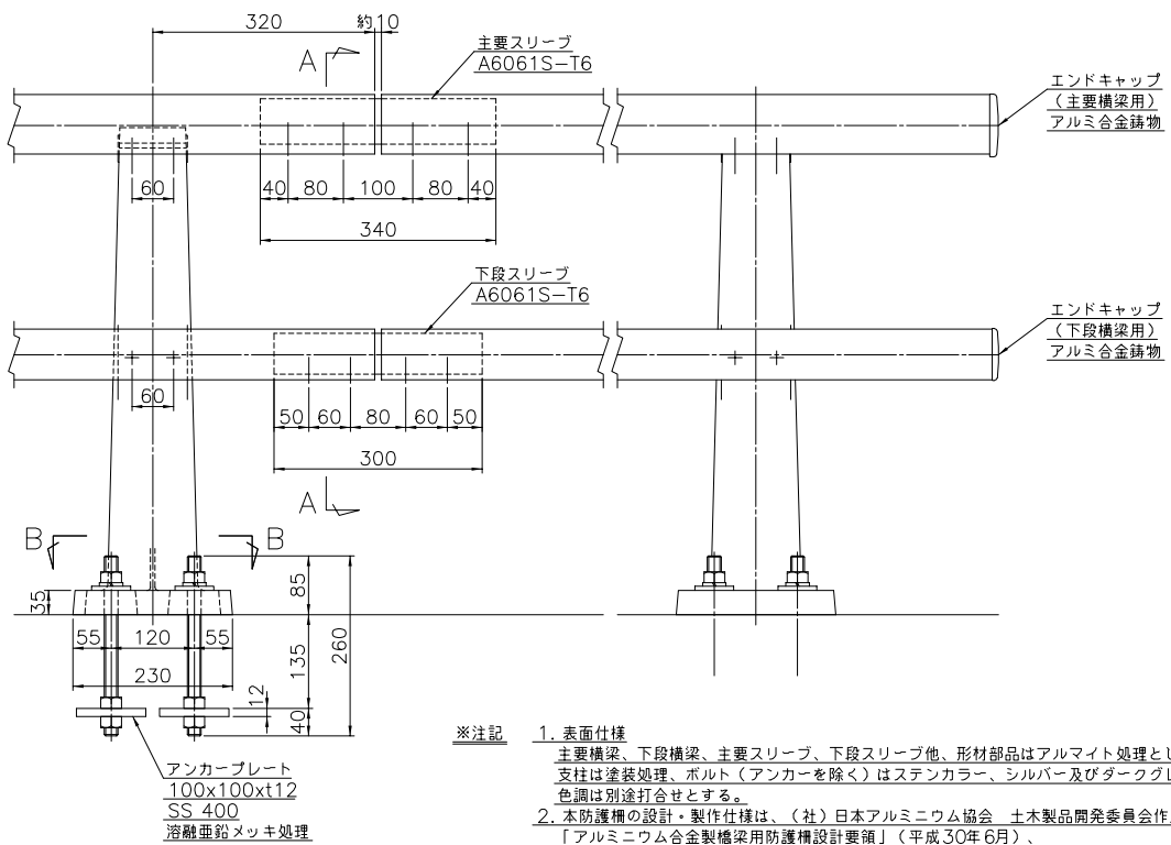
継手部
