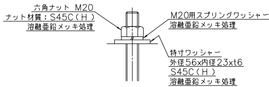
断面B-B
