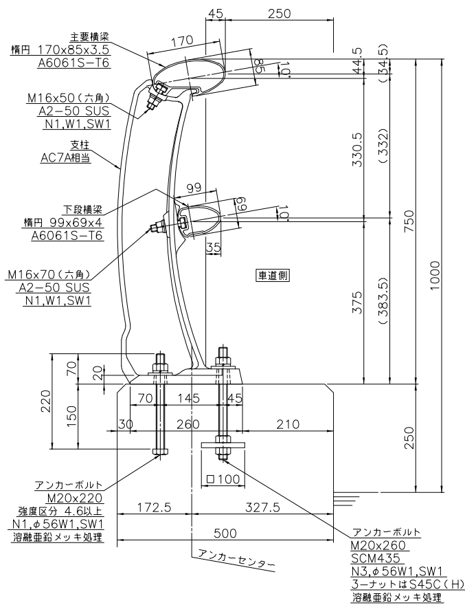
車両用防護柵取付詳細図 S=1/6
