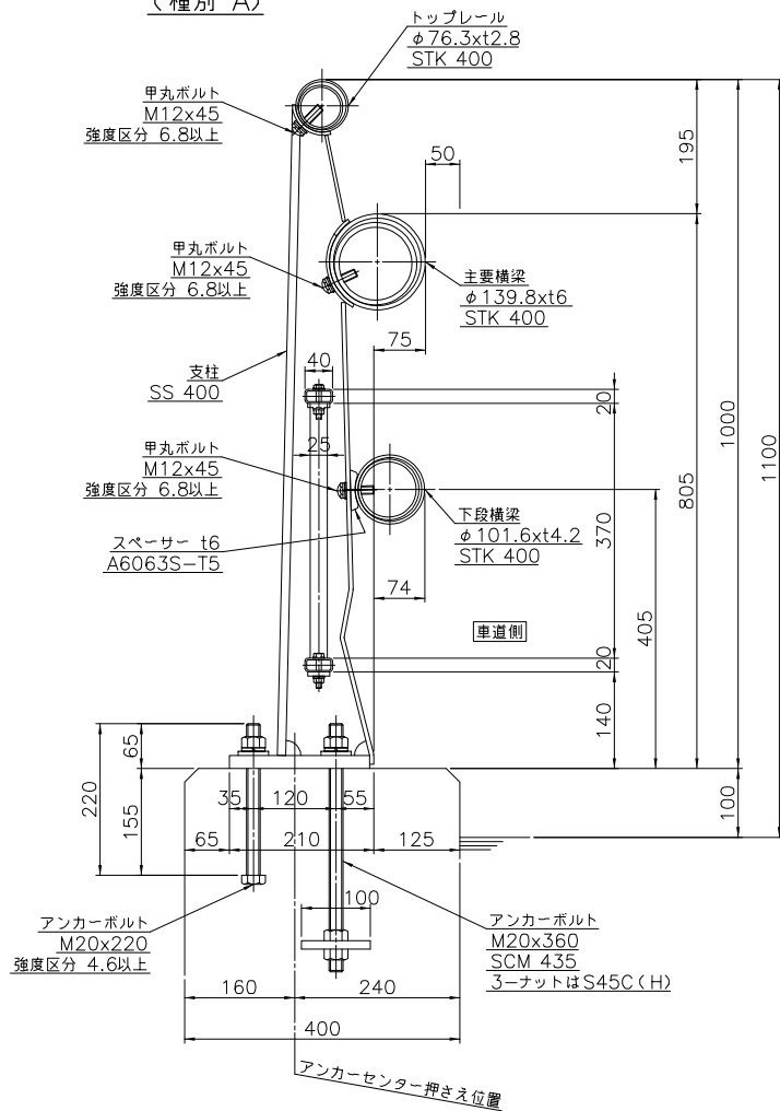
高欄兼用 車両用防護柵取付詳細図 S=1/6 (種別 A)
