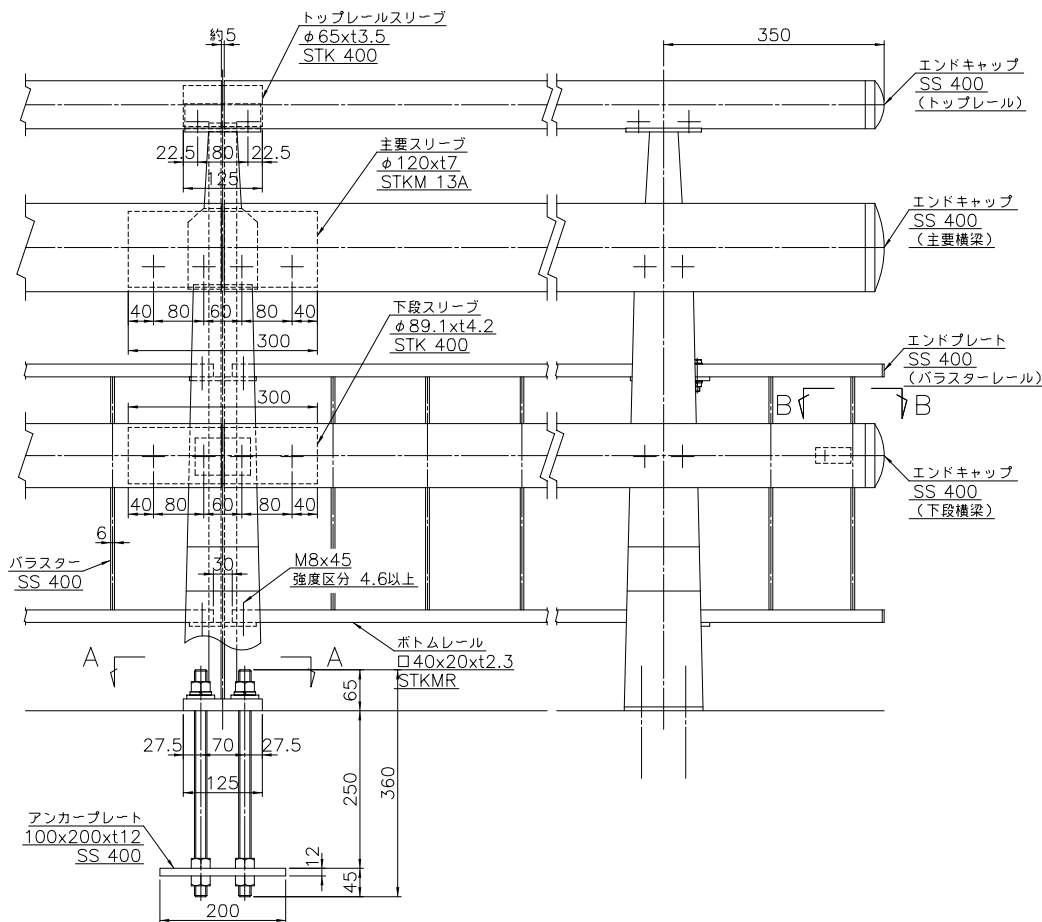
継手部
