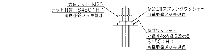
断面B-B
