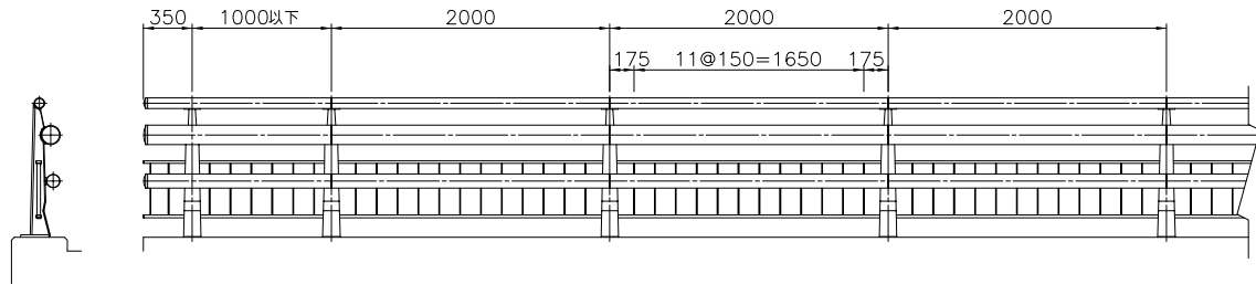
姿 図 S=1/30
