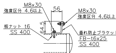
断面B-B
