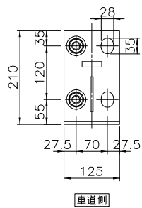
断面A-A
