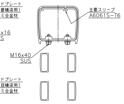
断面A-A
