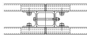
断面B-B
