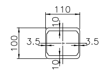
断面B-B
