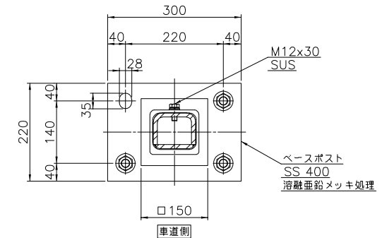
断面B-B
