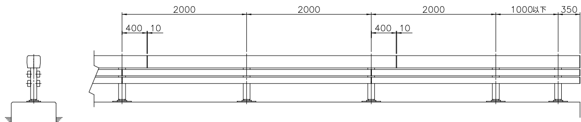
姿 図 S=1/30
