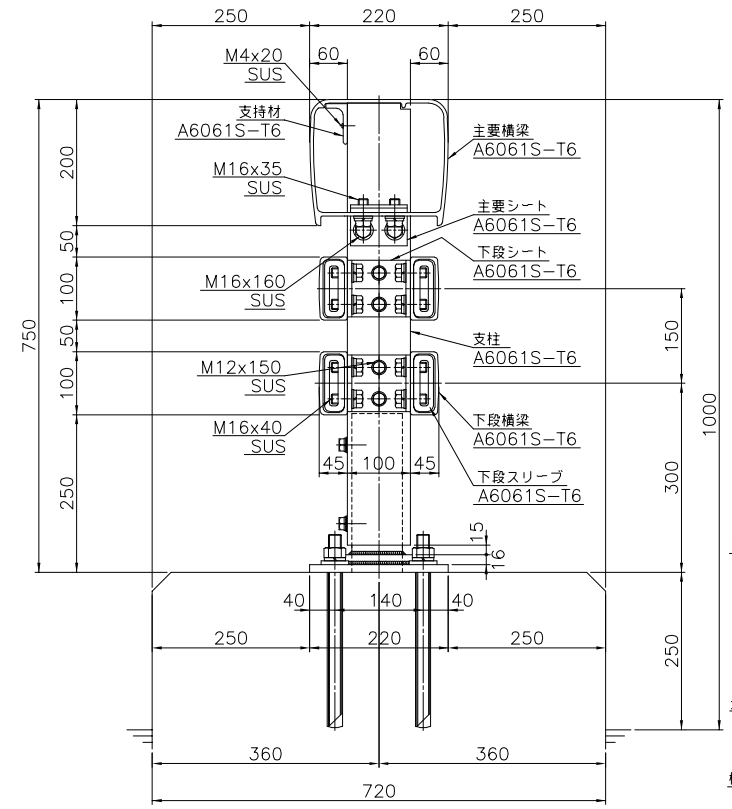
中央分離帯用 車両用防護柵取付詳細図
