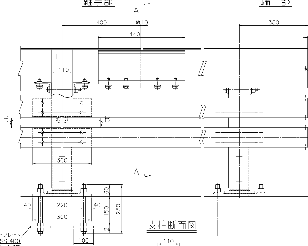
継手部
