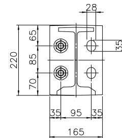
断面B-B
