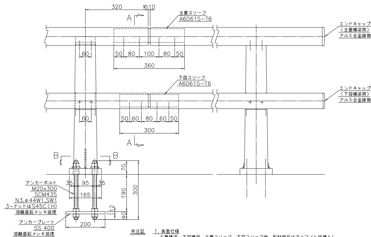
継手部
