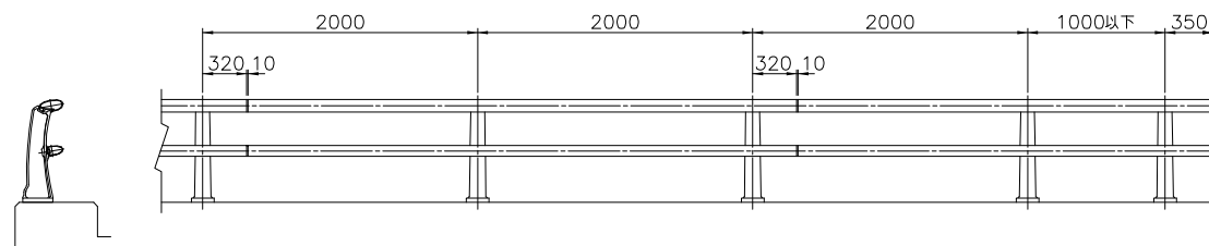
姿 図 S=1/30
