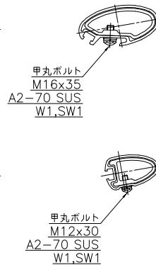
断面A-A
