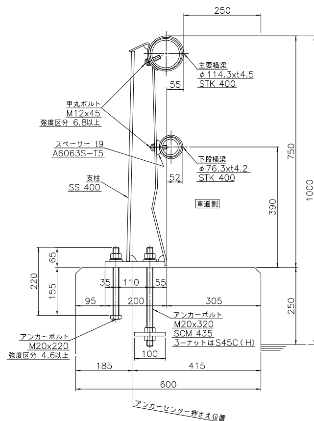
車両用防護柵取付詳細図 S=1/6 (種別 B)
