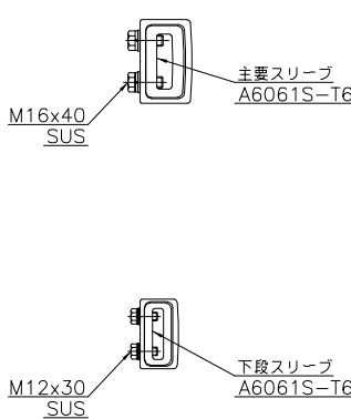
断面A-A
