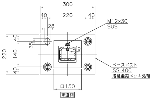
断面B-B
