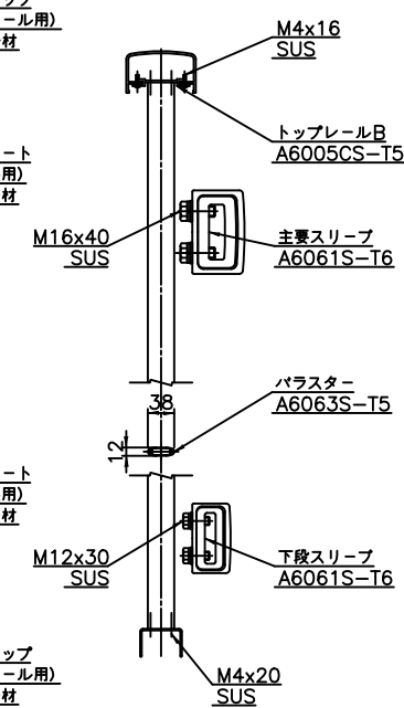
断面A-A
