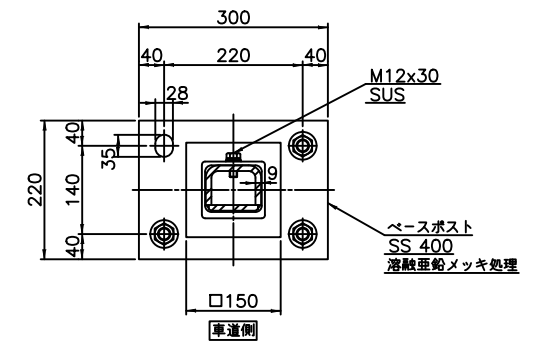
断面B-B
