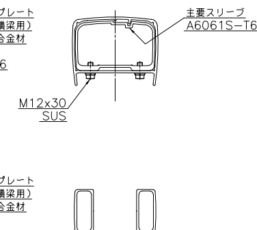
断面A-A
