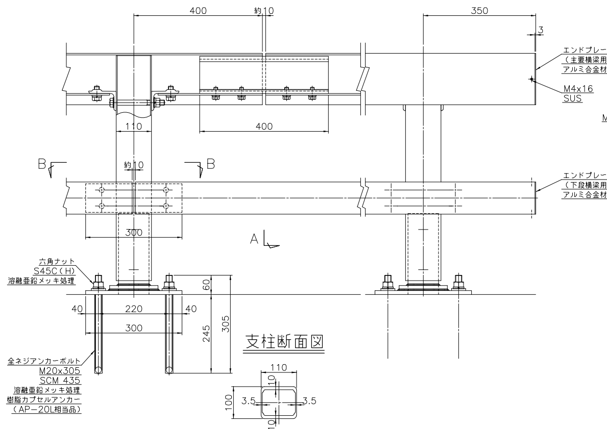
継手部
