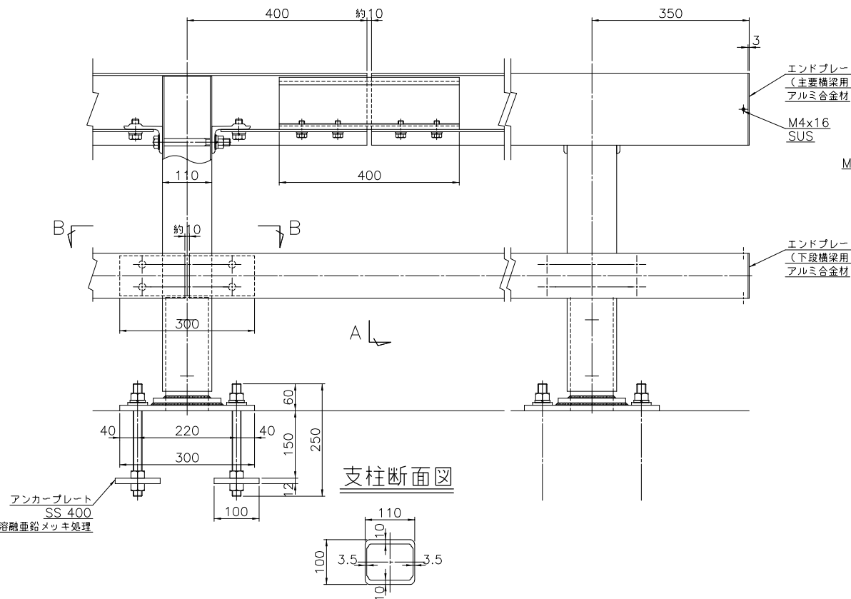
継手部
