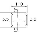
支柱断面図
