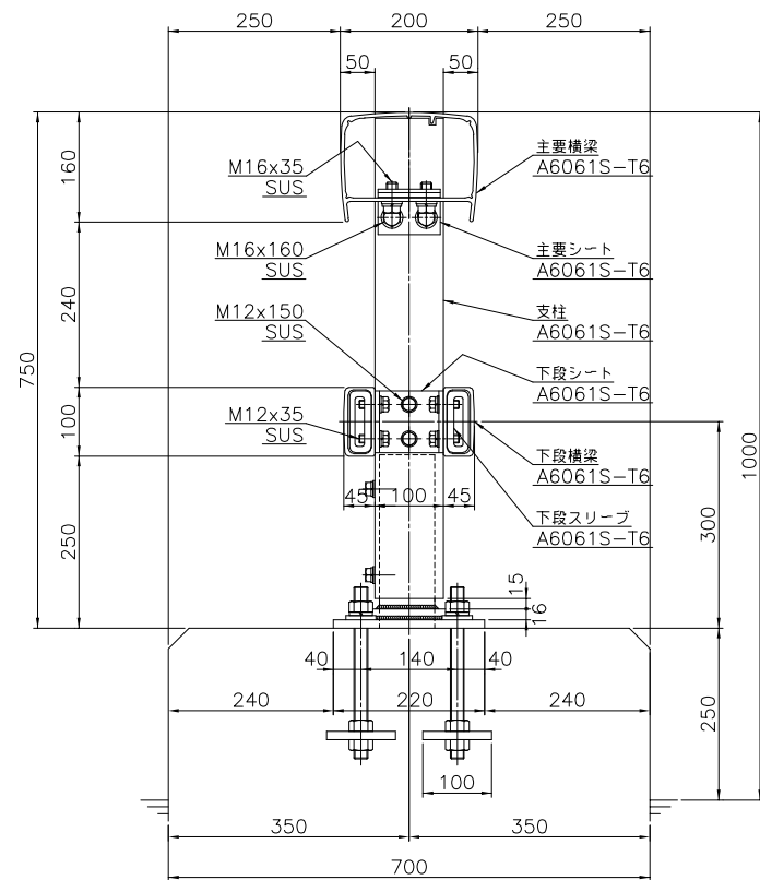
中央分離帯用 車両用防護柵取付詳細図 種別 C種 S=1/6
