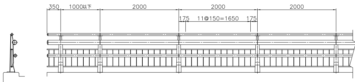
姿図 S=1/30
