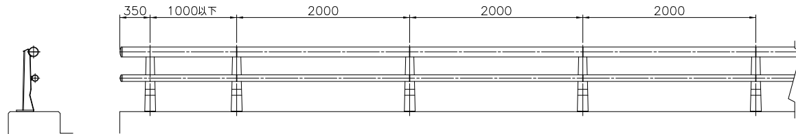
姿 図 S=1/30
