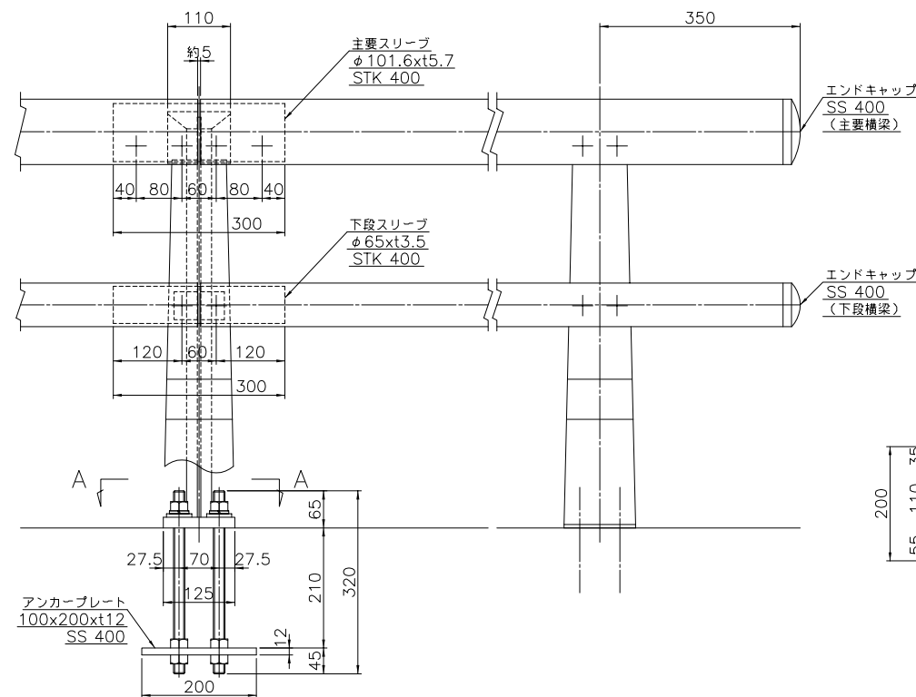
繼手部
