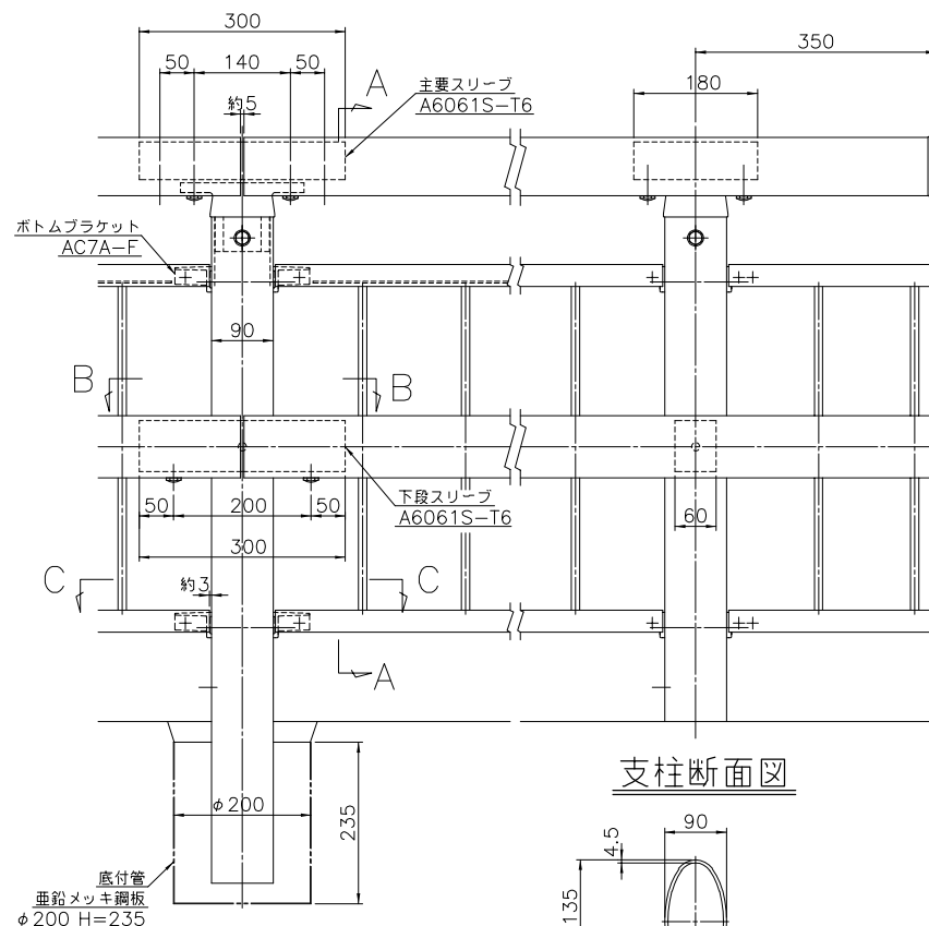
継手部
