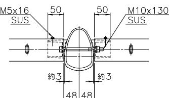
断面C-C
