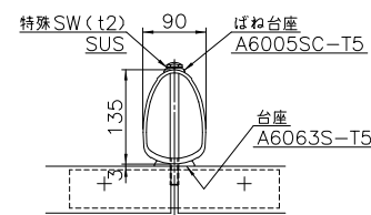
断面B-B
