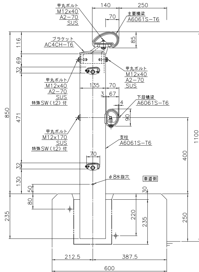
高欄兼用 車両防護柵取付詳細図 S=1/6 種別 C種
