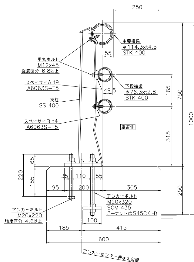
車両用防護柵取付詳細図 S=1/6 (種別 C)
