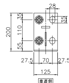
断面A-A
