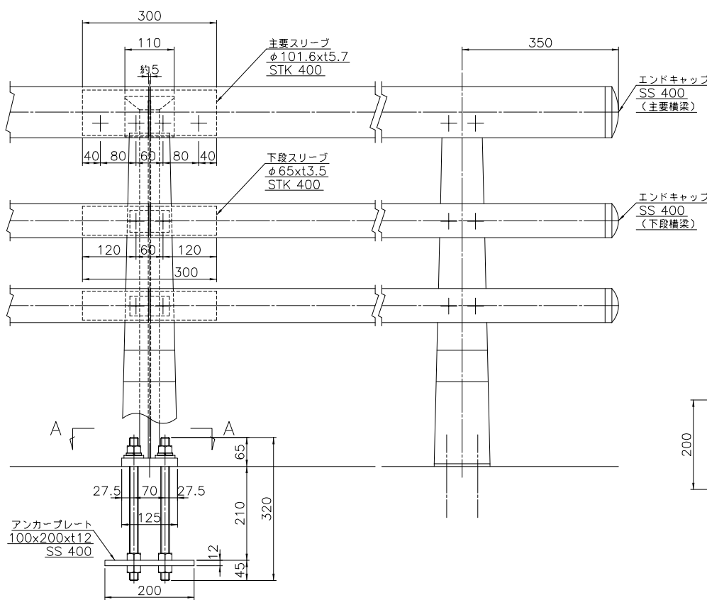
継手部
