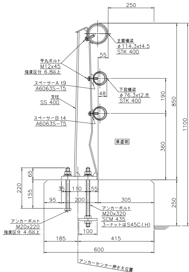
車両用防護柵取付詳細図 S=1/6
