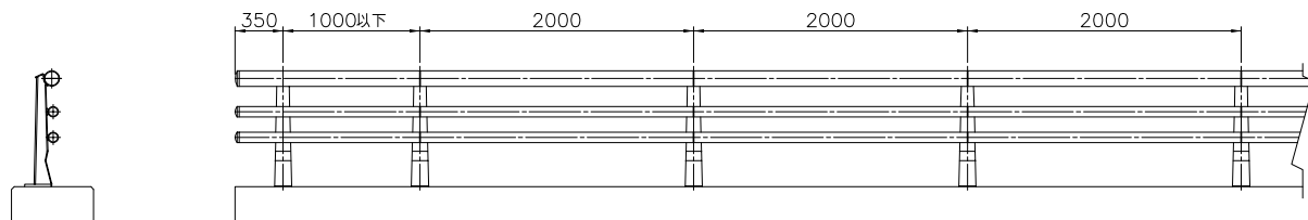
姿 図 S=1/30
