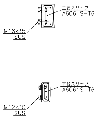
断面A-A
