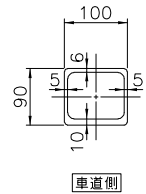
支柱断面図
