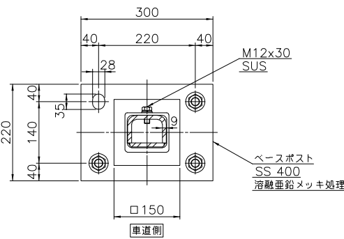
断面B-B
