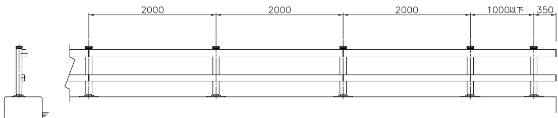
姿 図 S=1/30
