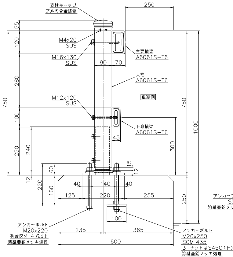
車両用防護柵取付詳細図
