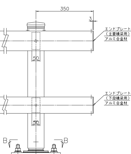
端 部
