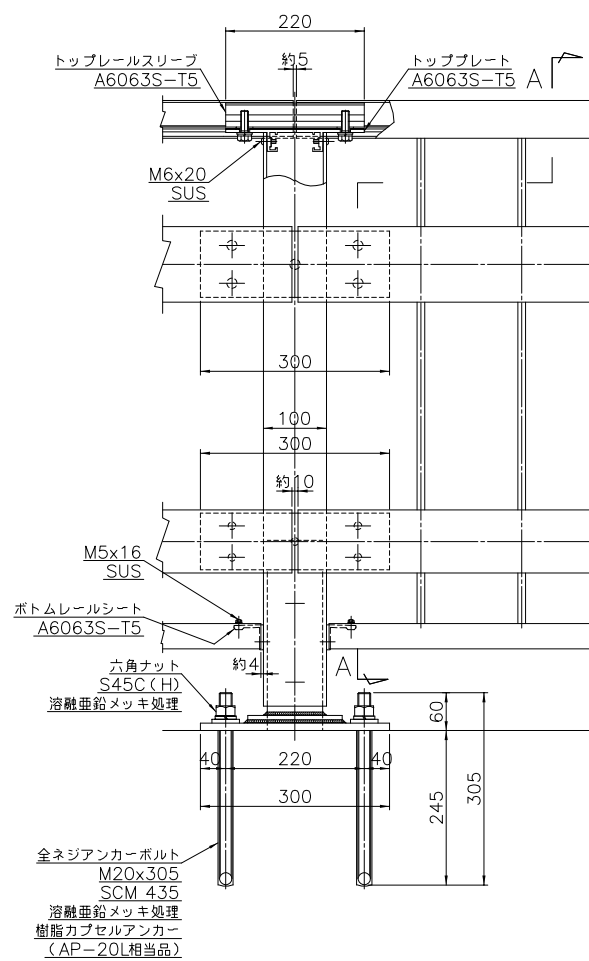
継手部
