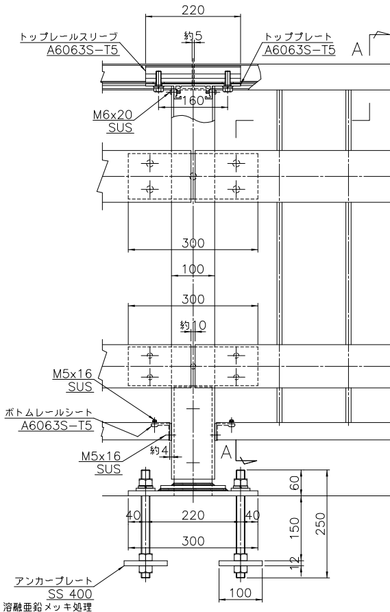
継手部
