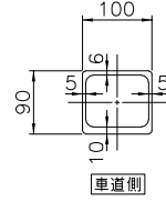
支柱断面図
