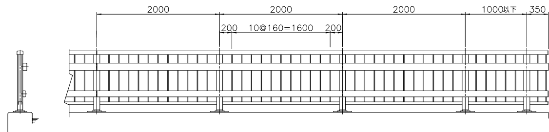
姿図 S=1/30
