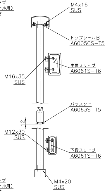
断面A-A
