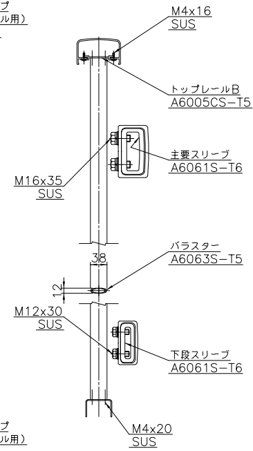
断面A-A
