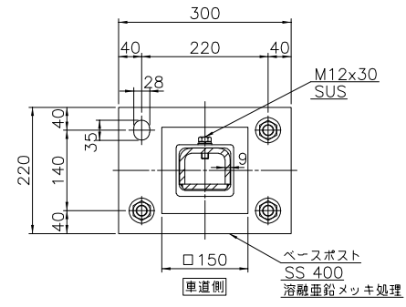
断面B-B
