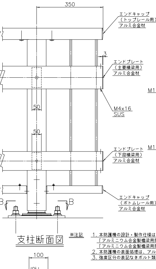
端部
