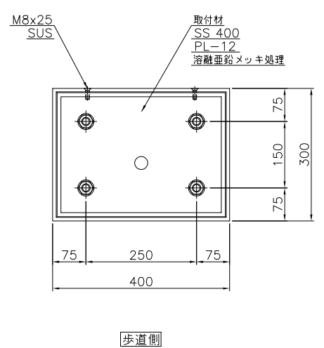
断面A-A
