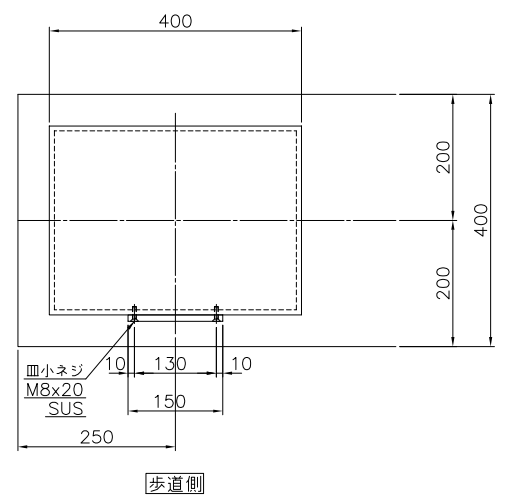
平面図 S=1/6
