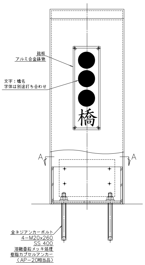
親柱取付詳細図 S=1/6
